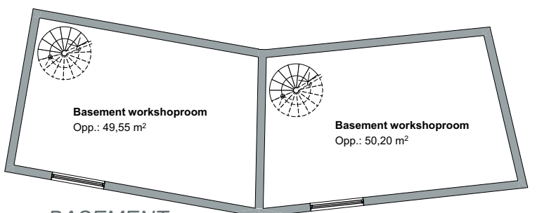
BASEMENT 1 : 200
